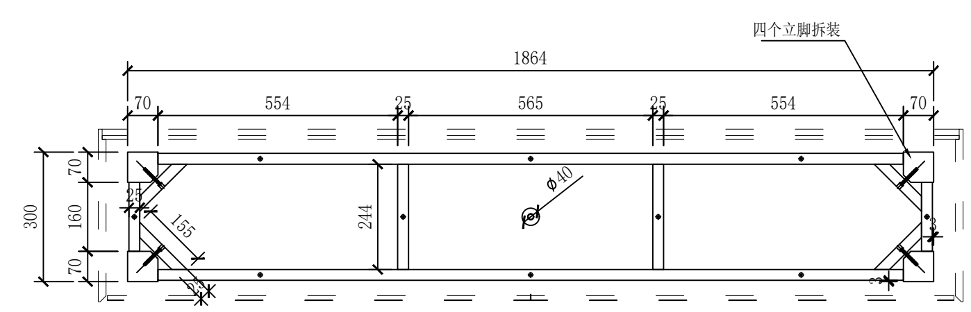
(C) 平面图
