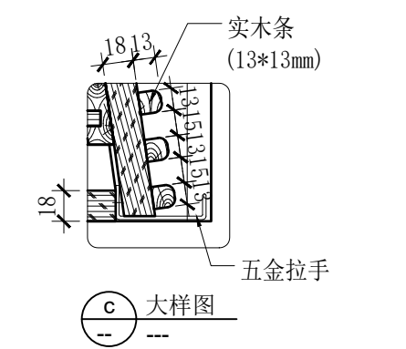
(b) 大样图
