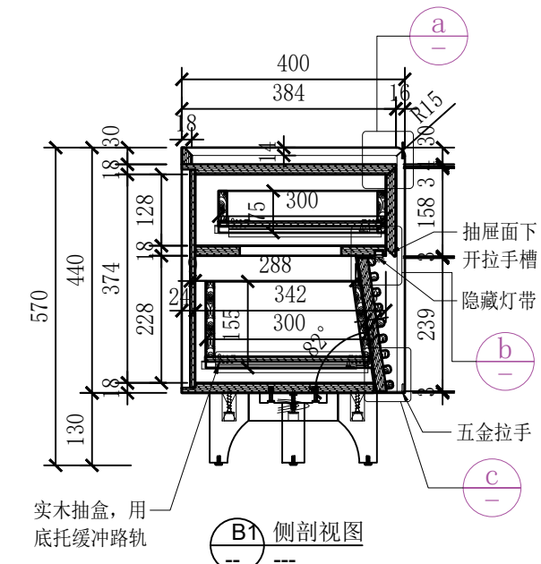
(B) 侧立面图
